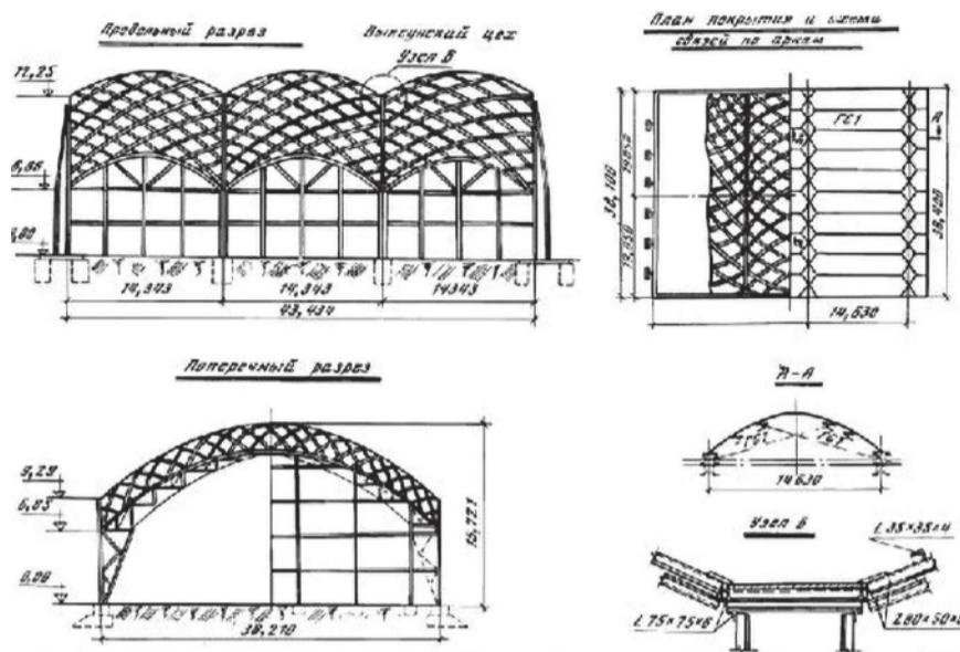
Чертеж перекрытия листопркатного цеха В.Г. Шухова на Выксунском металлургическом заводе
