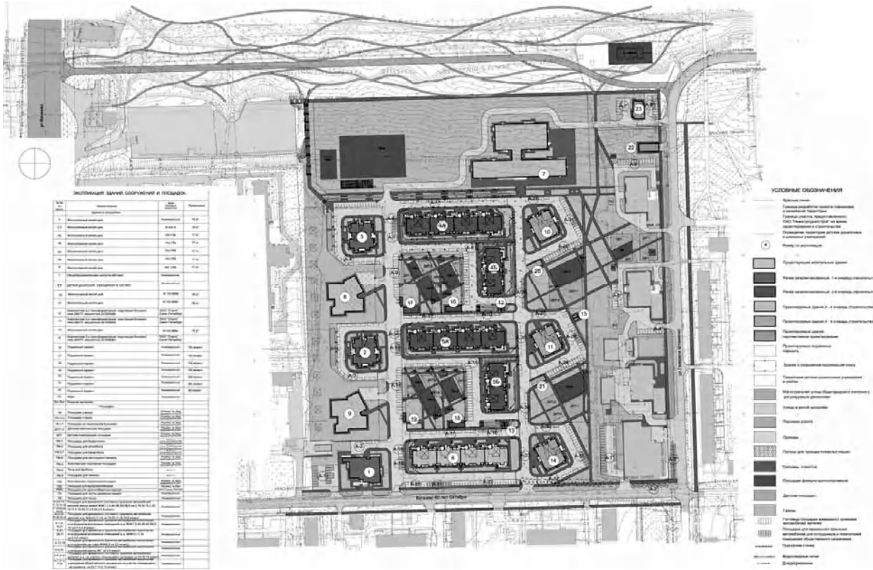
Чертеж планировки территории
